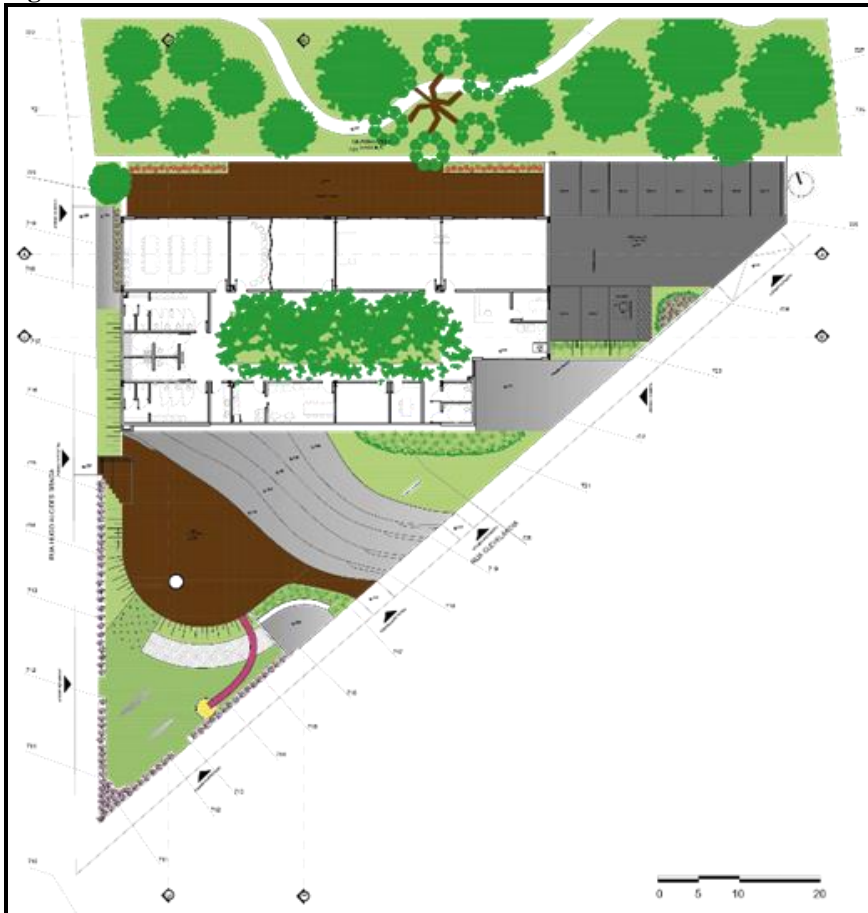
Figura 10: Planta baixa térreo.
