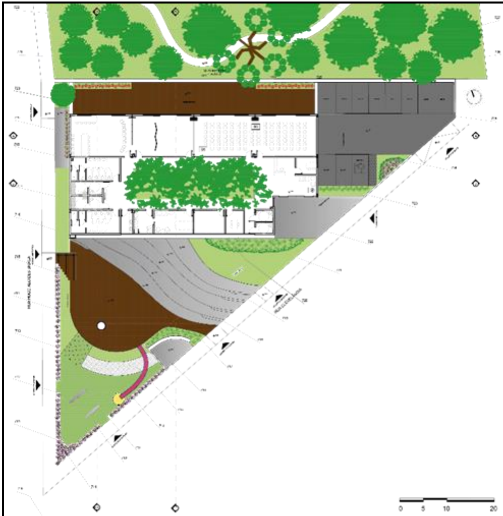
Figura 11: Planta baixa térreo com layout auditório.
